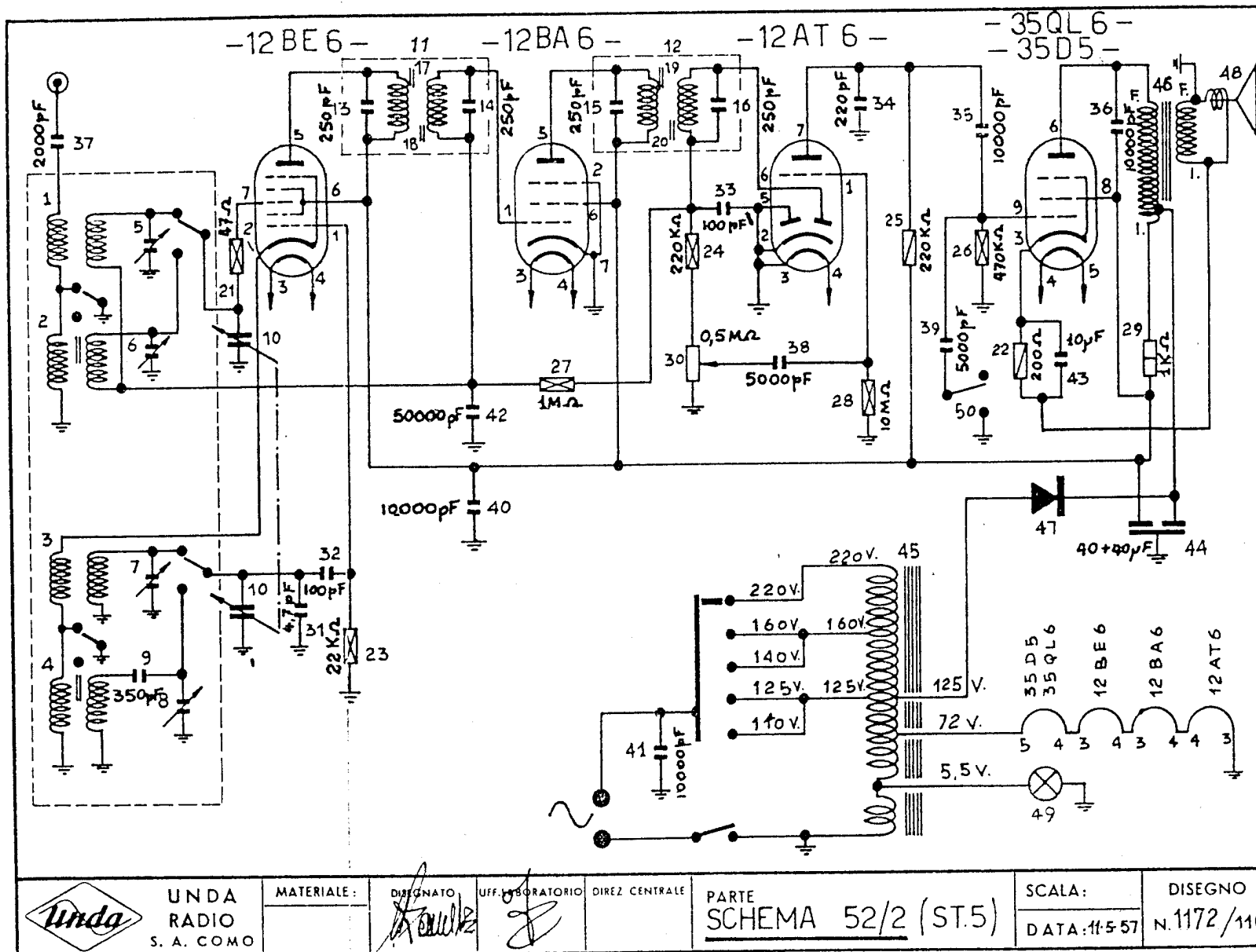
UNDA RADIO - Mod. 52/2. Apparecchio AM, di piccole dimensioni, con due gamme d'onda, OM da 182 a 580 m e OC da 15 a 51,5 m. Media frequenza a 467 kc/s. Potenza d'uscita 1,5 watt. Cons. 26 watt. Dimens. 240x166x124 mm. CC. 56 mA, CA 125 mA.
